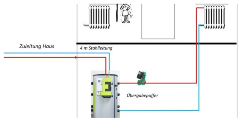
Abbildung 2 Ansicht Keller: Heizungssystem nach Anschluss der Nahwärme
