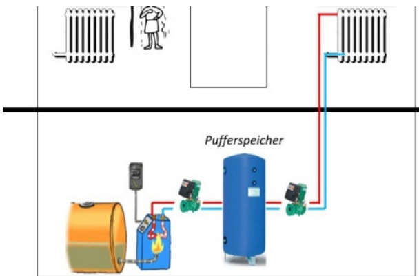
Abbildung 1 Ansicht Keller: Bestandsheizungssystem
