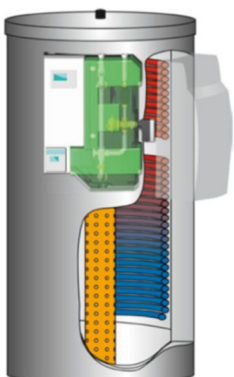
Abbildung 3 Nahwärmepufferspeicher
